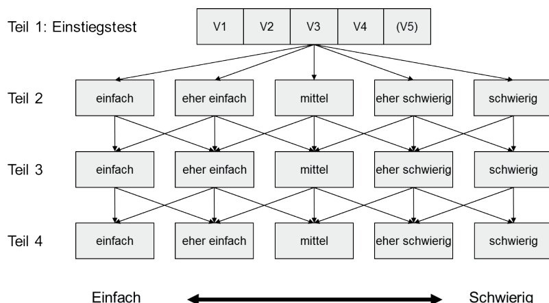
Abbildung 1: Aufbau adaptiver Online-Tests
